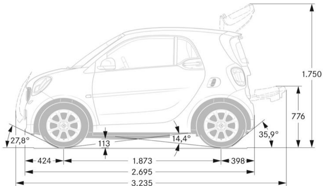
Размеры автомобиля типа smart
